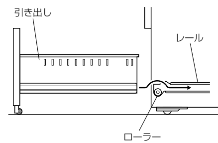
下段引き出しの入れかた
