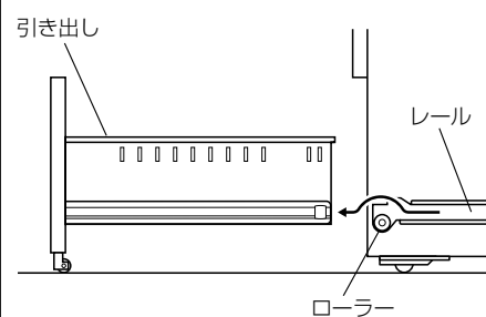
下段引き出しの抜きかた
