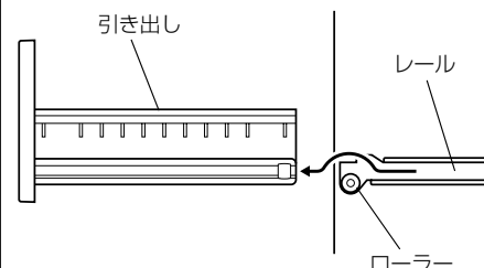
上・中段引き出しの抜きかた
